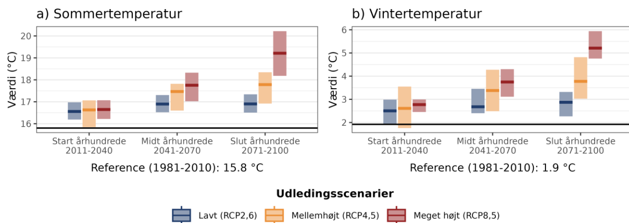
Figur 4. Fremtidens gennemsnitstemperatur for a) sommer (jun-aug) og b) vinter (dec-feb) under forskellige udledningsscenarier i Tønder Kommune. Den sorte linje viser værdien for referenceperioden (1981-2010).
