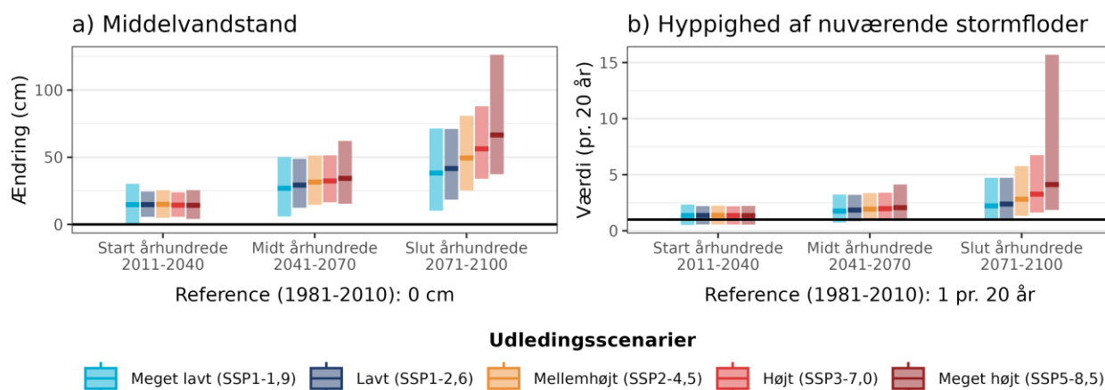
Figur 12. Fremtidens a) ændring i middelvandstand ift. referenceperioden 1981-2010 og b) hyppigheden af en nuværende 20-års stormflod for Vadehavskyst central under forskellige udledningsscenarioer. Den sorte linje viser værdien for referenceperioden (1981-2010). Bemærk også at denne indikator maksimalt viser 60 stormfloder per 20 år, selv hvis de beregnede værdier bliver endnu højere.
