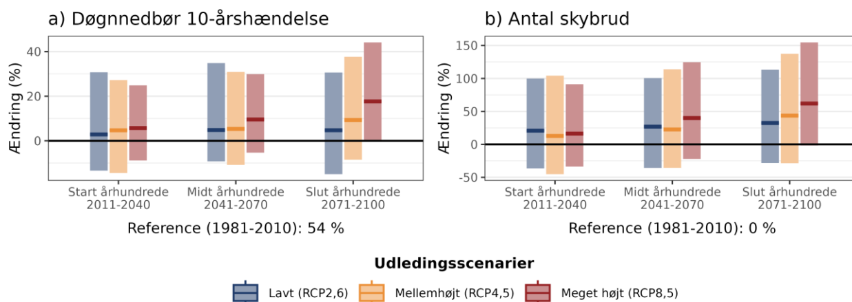
Figur 7. Procentvis ændring af a) 10-årshændelsen for døgnsnedbør og b) frekvensen af skybrud hen over året ift. 1981-2010 under forskellige udledningsscenarier i Tønder Kommune.
