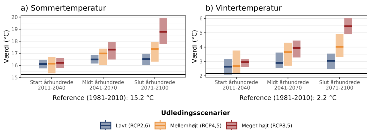
Figur 4. Fremtidens gennemsnitstemperatur for a) sommer (jun-aug) og b) vinter (dec-feb) under forskellige udledningsscenarier i Thisted Kommune. Den sorte linje viser værdien for referenceperioden (1981-2010).
