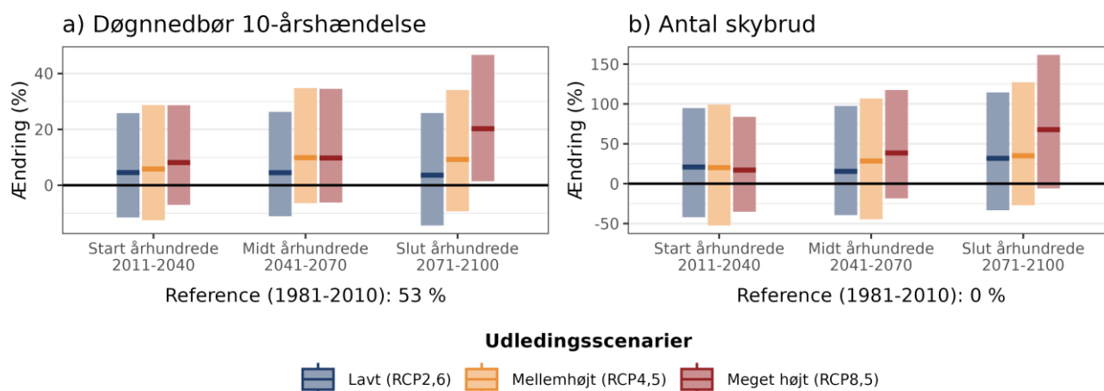
Figur 7. Procentvis ændring af a) 10-årshændelsen for døgnsnedbør og b) frekvensen af skybrud hen over året ift. 1981-2010 under forskellige udledningsscenarioer i Thisted Kommune.
