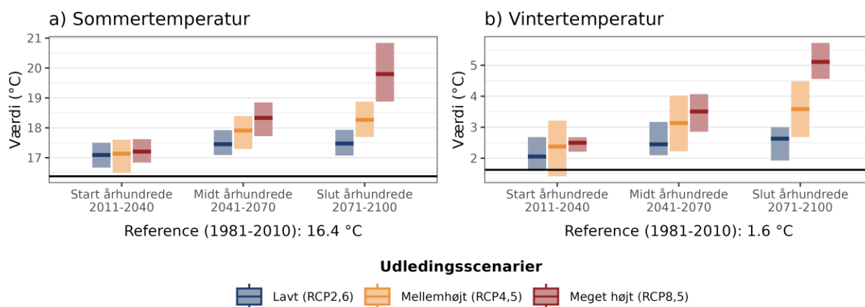
Figur 4. Fremtidens gennemsnitstemperatur for a) sommer (jun-aug) og b) vinter (dec-feb) under forskellige udledningsscenarier i Stevns Kommune. Den sorte linje viser værdien for referenceperioden (1981-2010).
