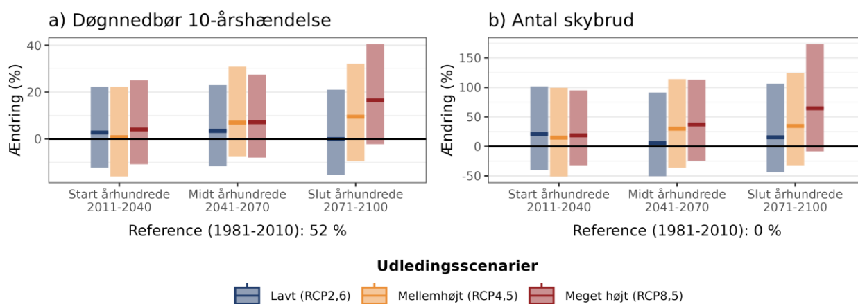
Figur 7. Procentvis ændring af a) 10-årshændelsen for døggnedbør og b) frekvensen af skybrud hen over året ift. 1981-2010 under forskellige udledningsscenarioer i Skanderborg Kommune.
