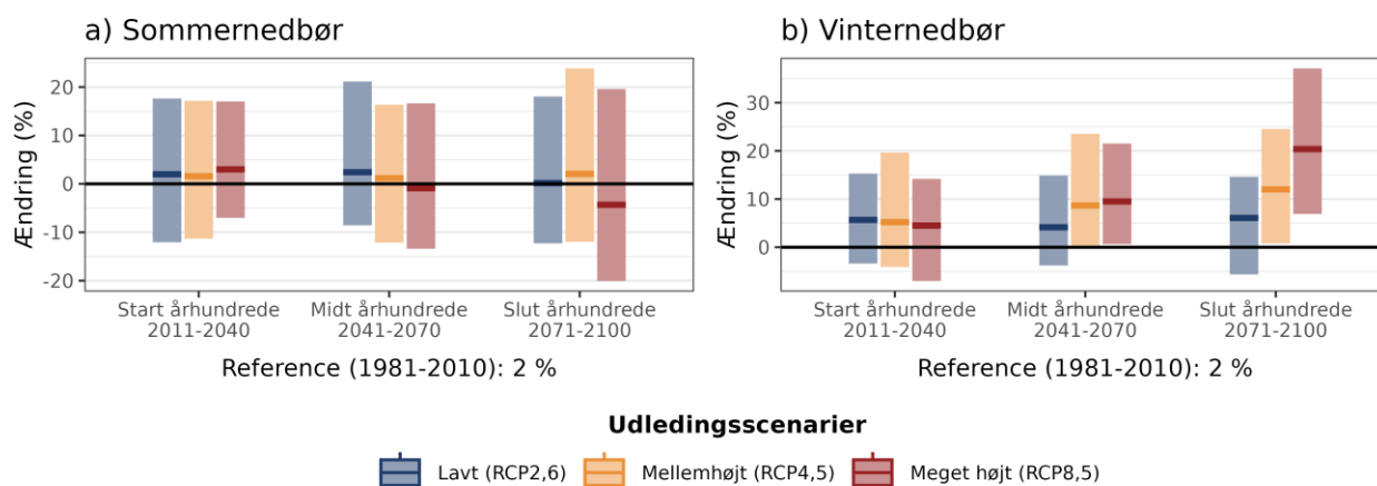
Figur 6. Procentvis ændring af middelnedbør a) om sommeren (jun-aug) og b) om vinteren (dec-feb) ift. referenceperioden 1981-2010 under forskellige udledningsscenarioer i Skanderborg Kommune.
