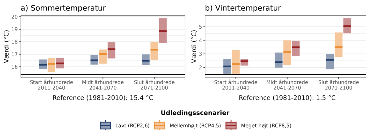
Figur 4. Fremtidens gennemsnitstemperatur for a) sommer (jun-aug) og b) vinter (dec-feb) under forskellige udledningsscenarier i Skanderborg Kommune. Den sorte linje viser værdien for referenceperioden (1981-2010).
