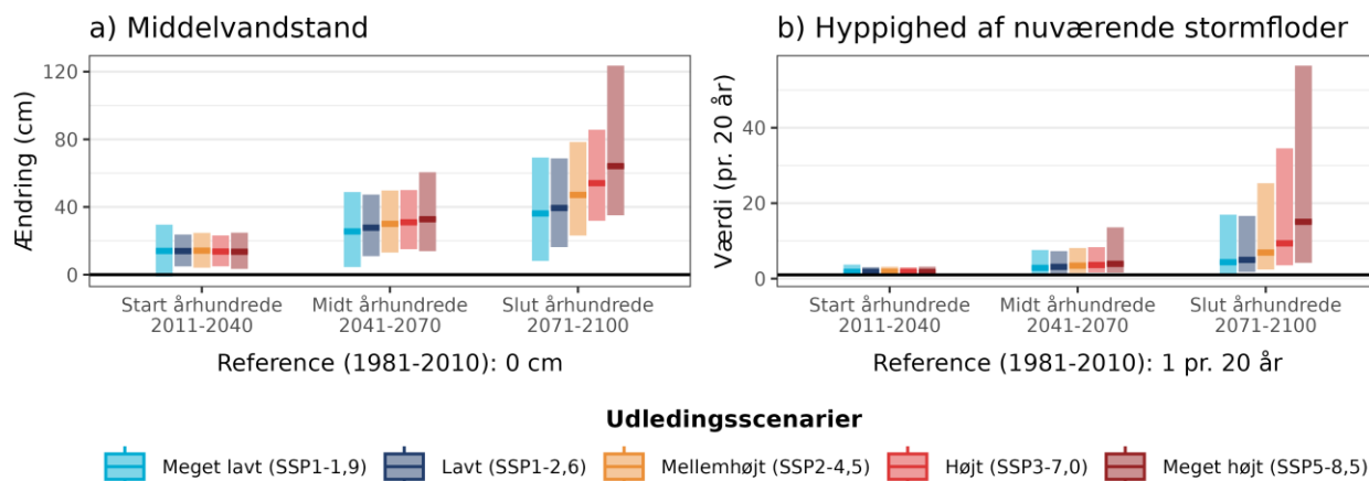
Figur 10. Fremtidens a) ændring i middelvandstand ift. referenceperioden 1981-2010 og b) hyppigheden af en nuværende 20-års stormflod for Vestkyst central under forskellige udledningsscenarier. Den sorte linje viser værdien for referenceperioden (1981-2010). Bemærk også at denne indikator maksimalt viser 60 stormfloder per 20 år, selv hvis de beregnede værdier bliver endnu højere.
