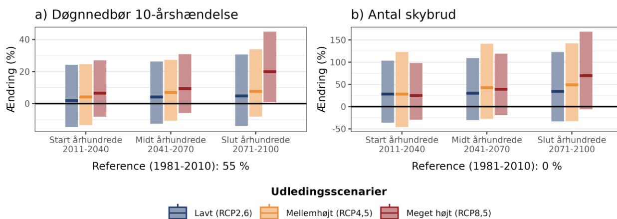
Figur 7. Procentvis ændring af a) 10-årshændelsen for døggnedbør og b) frekvensen af skybrud hen over året ift. 1981-2010 under forskellige udledningsscenarier i Ringkøbing-Skjern Kommune.
