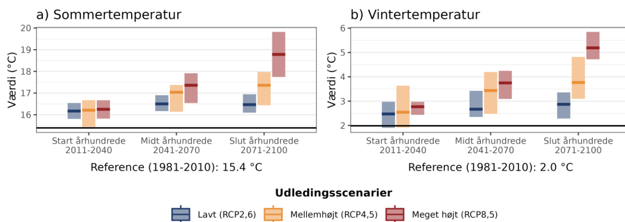
Figur 4. Fremtidens gennemsnitstemperatur for a) sommer (jun-aug) og b) vinter (dec-feb) under forskellige udledningsscenarier i Ringkøbing-Skjern Kommune. Den sorte linje viser værdien for referenceperioden (1981-2010).
