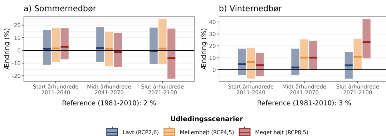
Figur 6. Procentvis ændring af middelnedbør a) om sommeren (jun-aug) og b) om vinteren (dec-feb) ift. referenceperioden 1981-2010 under forskellige udledningsscenarier i Ringkøbing-Skjern Kommune.
