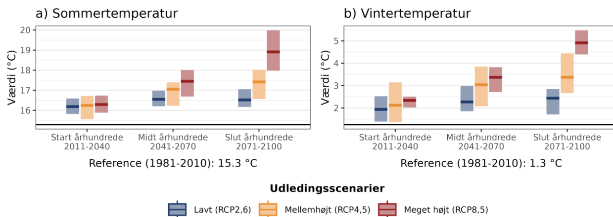
Figur 4. Fremtidens gennemsnitstemperatur for a) sommer (jun-aug) og b) vinter (dec-feb) under forskellige udledningsscenarier i Randers Kommune. Den sorte linje viser værdien for referenceperioden (1981-2010).
