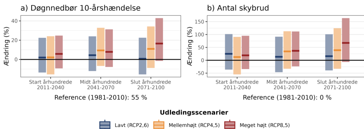
Figur 7. Procentvis ændring af a) 10-årshændelsen for døgnsnedbør og b) frekvensen af skybrud hen over året ift. 1981-2010 under forskellige udledningsscenarioer i Randers Kommune.
