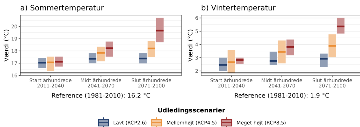
Figur 4. Fremtidens gennemsnitstemperatur for a) sommer (jun-aug) og b) vinter (dec-feb) under forskellige udledningsscenarier i Nyborg Kommune. Den sorte linje viser værdien for referenceperioden (1981-2010).
