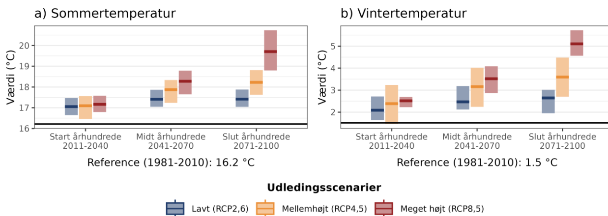
Figur 4. Fremtidens gennemsnitstemperatur for a) sommer (jun-aug) og b) vinter (dec-feb) under forskellige udledningsscenarier i Næstved Kommune. Den sorte linje viser værdien for referenceperioden (1981-2010).
