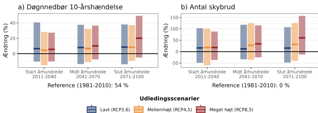
Figur 7. Procentvis ændring af a) 10-årshændelsen for døgnsnedbør og b) frekvensen af skybrud hen over året ift. 1981-2010 under forskellige udledningsscenarier i Næstved Kommune.
