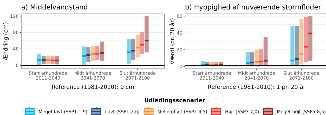
Figur 10. Fremtidens a) ændring i middelvandstand ift. referenceperioden 1981-2010 og b) hyppigheden af en nuværende 20-års stormflod for Smålandsfarvandet under forskellige udledningsscenarioer. Den sorte linje viser værdien for referenceperioden (1981-2010). Bemærk også at denne indikator maksimalt viser 60 stormfloder per 20 år, selv hvis de beregnede værdier bliver endnu højere.
