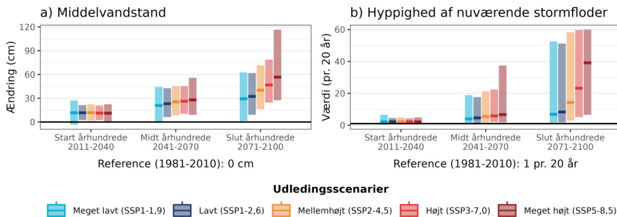
Figur 14. Fremtidens a) ændring i middelvandstand ift. referenceperioden 1981-2010 og b) hyppigheden af en nuværende 20-års stormflod for Limfjorden ved Thisted under forskellige udledningsscenarier. Den sorte linje viser værdien for referenceperioden (1981-2010). Bemærk også at denne indikator maksimalt viser 60 stormfloder per 20 år, selv hvis de beregnede værdier bliver endnu højere.
