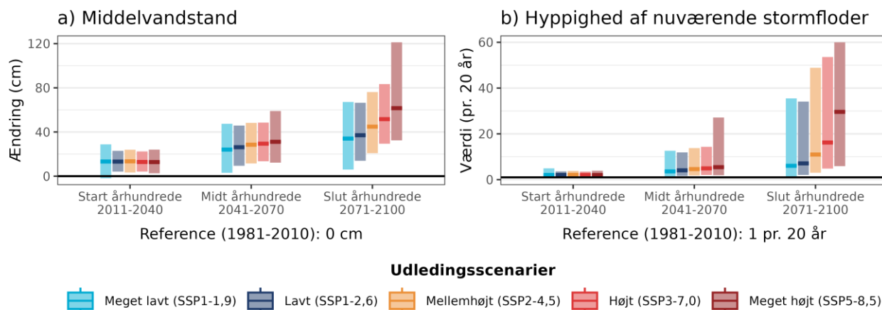
Figur 12. Fremtidens a) ændring i middelvandstand ift. referenceperioden 1981-2010 og b) hyppigheden af en nuværende 20-års stormflod for Limfjorden ved Lemvig under forskellige udledningsscenarier. Den sorte linje viser værdien for referenceperioden (1981-2010). Bemærk også at denne indikator maksimalt viser 60 stormfloder per 20 år, selv hvis de beregnede værdier bliver endnu højere.
