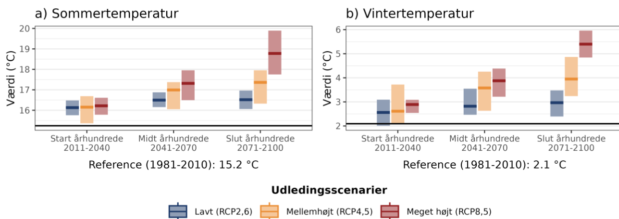
Figur 4. Fremtidens gennemsnitstemperatur for a) sommer (jun-aug) og b) vinter (dec-feb) under forskellige udledningsscenarier i Morsø Kommune. Den sorte linje viser værdien for referenceperioden (1981-2010).
