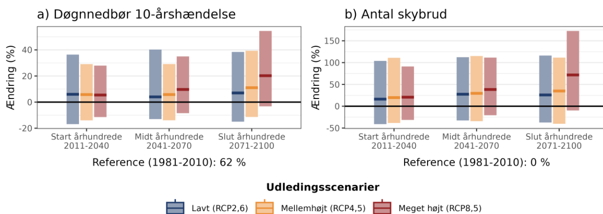
Figur 7. Procentvis ændring af a) 10-årshændelsen for døggnedbør og b) frekvensen af skybrud hen over året ift. 1981-2010 under forskellige udledningsscenarioer i Lyngby-Taarbæk Kommune.
