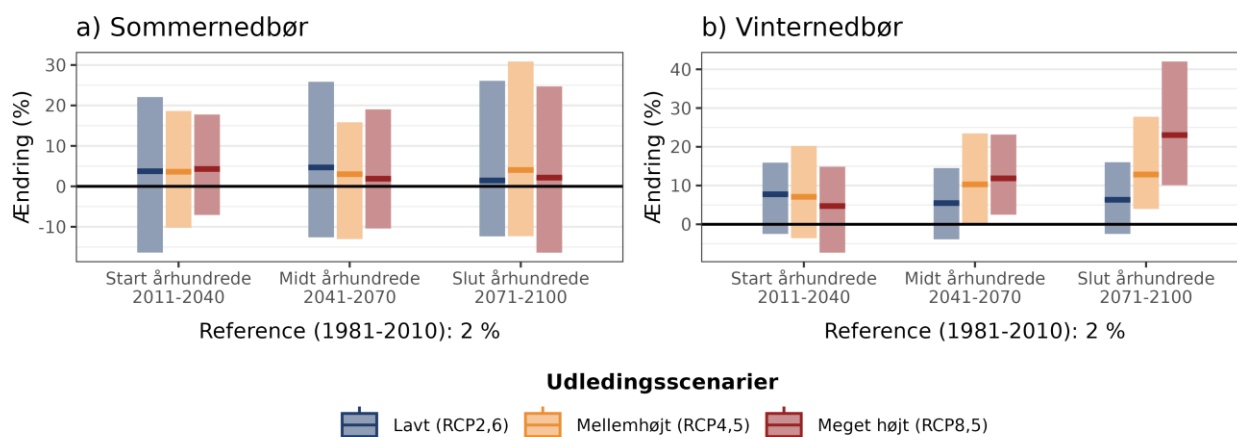
Figur 6. Procentvis ændring af middelnedbør a) om sommeren (jun-aug) og b) om vinteren (dec-feb) ift. referenceperioden 1981-2010 under forskellige udledningsscenarioer i Lyngby-Taarbæk Kommune.
