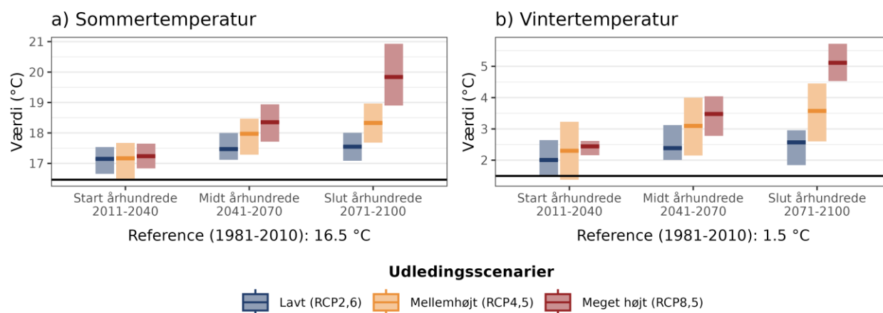
Figur 4. Fremtidens gennemsnitstemperatur for a) sommer (jun-aug) og b) vinter (dec-feb) under forskellige udledningsscenarier i Lyngby-Taarbæk Kommune. Den sorte linje viser værdien for referenceperioden (1981-2010).
