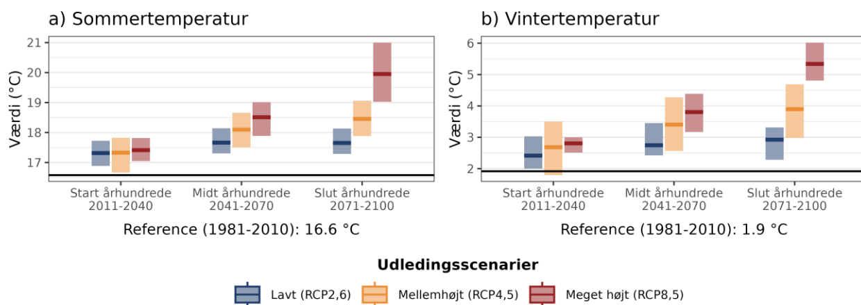
Figur 4. Fremtidens gennemsnitstemperatur for a) sommer (jun-aug) og b) vinter (dec-feb) under forskellige udledningsscenarier i Lolland Kommune. Den sorte linje viser værdien for referenceperioden (1981-2010).
