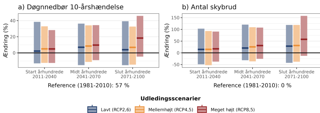
Figur 7. Procentvis ændring af a) 10-årshændelsen for døgnnedbør og b) frekvensen af skybrud hen over året ift. 1981-2010 under forskellige udledningsscenarier i Lolland Kommune.
