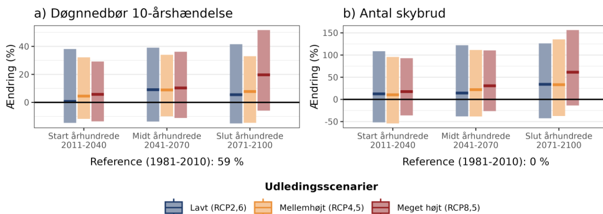
Figur 7. Procentvis ændring af a) 10-årshændelsen for døgnsnedbør og b) frekvensen af skybrud hen over året ift. 1981-2010 under forskellige udledningsscenarier i Langeland Kommune.
