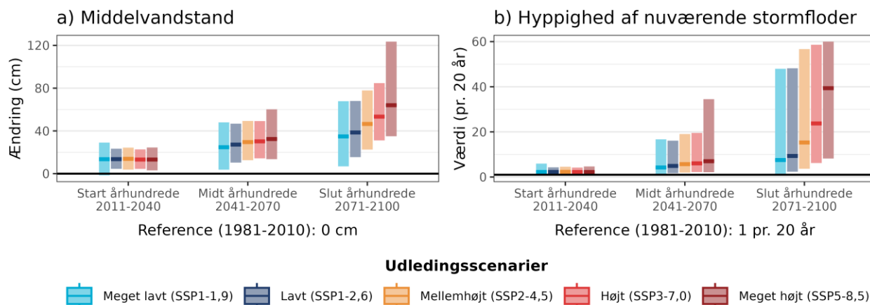
Figur 14. Fremtidens a) ændring i middelvandstand ift. referenceperioden 1981-2010 og b) hyppigheden af en nuværende 20-års stormflod for Femern Bælt under forskellige udledningsscenarioer. Den sorte linje viser værdien for referenceperioden (1981-2010). Bemærk også at denne indikator maksimalt viser 60 stormfloder per 20 år, selv hvis de beregnede værdier bliver endnu højere.
