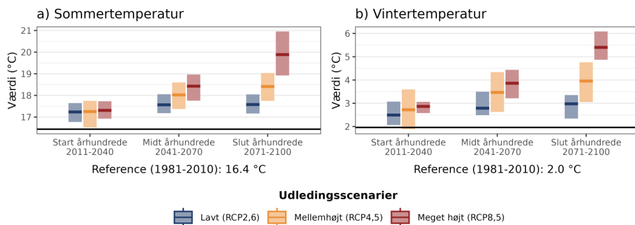
Figur 4. Fremtidens gennemsnitstemperatur for a) sommer (jun-aug) og b) vinter (dec-feb) under forskellige udledningsscenarier i Langeland Kommune. Den sorte linje viser værdien for referenceperioden (1981-2010).
