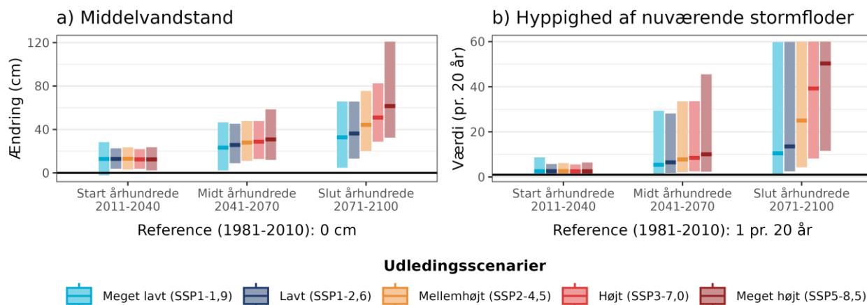
Figur 12. Fremtidens a) ændring i middelvandstand ift. referenceperioden 1981-2010 og b) hyppigheden af en nuværende 20-års stormflod for Storebælt Sydvest under forskellige udledningsscenarier. Den sorte linje viser værdien for referenceperioden (1981-2010). Bemærk også at denne indikator maksimalt viser 60 stormfloder per 20 år, selv hvis de beregnede værdier bliver endnu højere.
