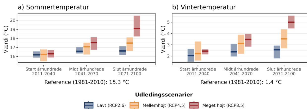
Figur 4. Fremtidens gennemsnitstemperatur for a) sommer (jun-aug) og b) vinter (dec-feb) under forskellige udledningsscenarier i Læsø Kommune. Den sorte linje viser værdien for referenceperioden (1981-2010).
