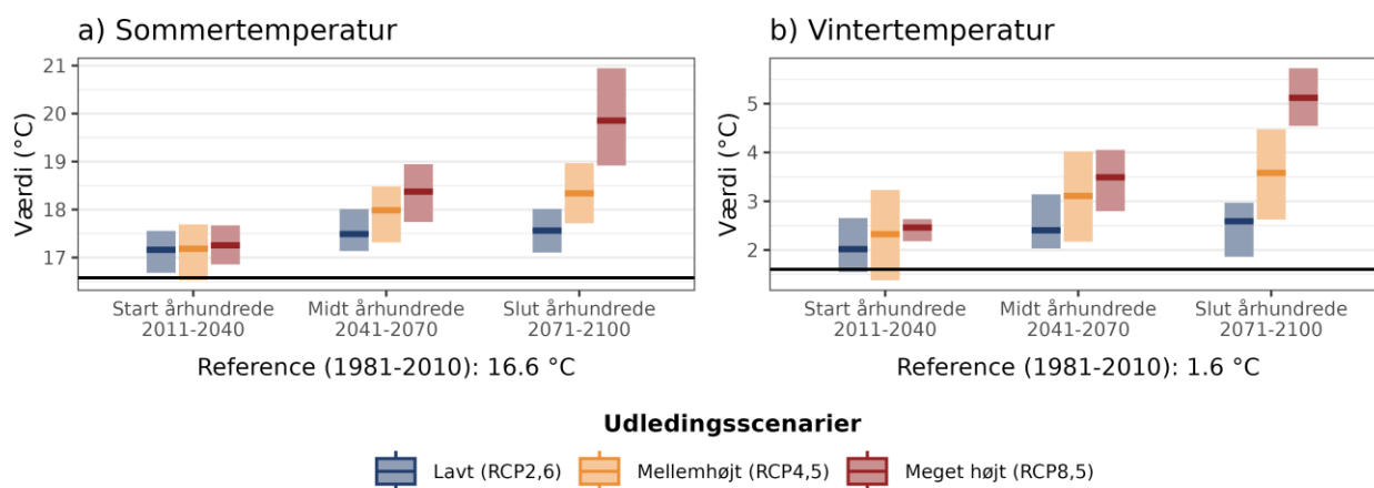
Figur 4. Fremtidens gennemsnitstemperatur for a) sommer (jun-aug) og b) vinter (dec-feb) under forskellige udledningsscenarier i Københavns Kommune. Den sorte linje viser værdien for referenceperioden (1981-2010).
