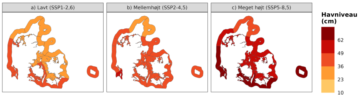
Figur 9. Ændring mellem 1981-2010 og fremtidsperioden 2071-2100 i middelvandstand (cm) for hele Danmark i et a) lavt, b) mellemhøjt og c) højt udledningsscenarie.
