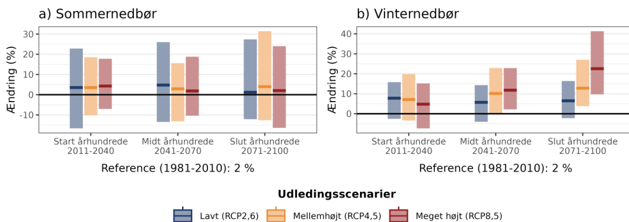
Figur 6. Procentvis ændring af middelnedbør a) om sommeren (jun-aug) og b) om vinteren (dec-feb) ift. referenceperioden 1981-2010 under forskellige udledningsscenarier i Københavns Kommune.
