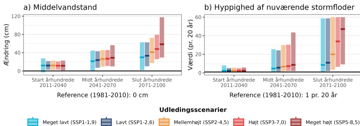
Figur 12. Fremtidens a) ændring i middelvandstand ift. referenceperioden 1981-2010 og b) hyppigheden af en nuværende 20-års stormflod for Køge Bugt under forskellige udledningsscenarier. Den sorte linje viser værdien for referenceperioden (1981-2010). Bemærk også at denne indikator maksimalt viser 60 stormfloder per 20 år, selv hvis de beregnede værdier bliver endnu højere.
