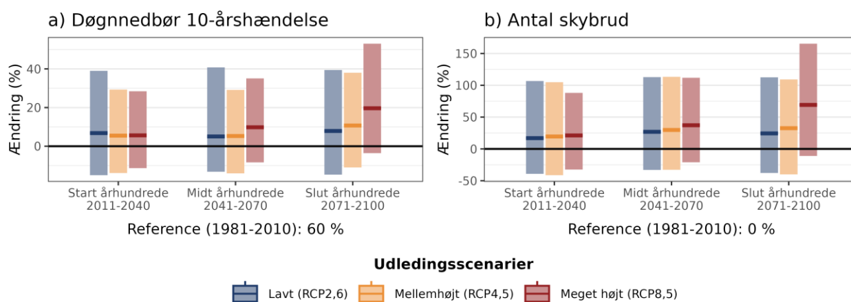
Figur 7. Procentvis ændring af a) 10-årshændelsen for døggnedbør og b) frekvensen af skybrud hen over året ift. 1981-2010 under forskellige udledningsscenarier i Københavns Kommune.
