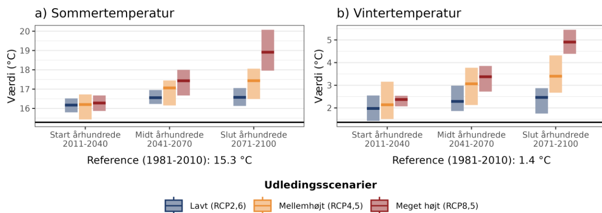
Figur 4. Fremtidens gennemsnitstemperatur for a) sommer (jun-aug) og b) vinter (dec-feb) under forskellige udledningsscenarier i Hjørring Kommune. Den sorte linje viser værdien for referenceperioden (1981-2010).
