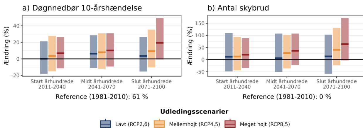
Figur 7. Procentvis ændring af a) 10-årshændelsen for døgnnedbør og b) frekvensen af skybrud hen over året ift. 1981-2010 under forskellige udledningsscenarier i Hjørring Kommune.
