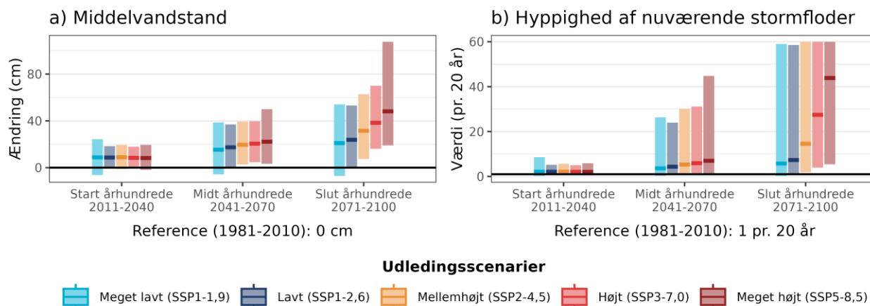
Figur 10. Fremtidens a) ændring i middelvandstand ift. referenceperioden 1981-2010 og b) hyppigheden af en nuværende 20-års stormflod for Skagerrakkyst nordlig under forskellige udledningsscenarier. Den sorte linje viser værdien for referenceperioden (1981-2010). Bemærk også at denne indikator maksimalt viser 60 stormfloder per 20 år, selv hvis de beregnede værdier bliver endnu højere.
