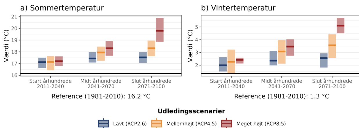
Figur 4. Fremtidens gennemsnitstemperatur for a) sommer (jun-aug) og b) vinter (dec-feb) under forskellige udledningsscenarier i Helsingør Kommune. Den sorte linje viser værdien for referenceperioden (1981-2010).
