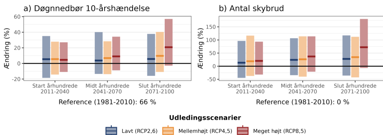
Figur 7. Procentvis ændring af a) 10-årshændelsen for døgnnedbør og b) frekvensen af skybrud hen over året ift. 1981-2010 under forskellige udledningsscenarier i Helsingør Kommune.
