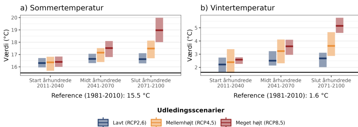
Figur 4. Fremtidens gennemsnitstemperatur for a) sommer (jun-aug) og b) vinter (dec-feb) under forskellige udledningsscenarier i Hedensted Kommune. Den sorte linje viser værdien for referenceperioden (1981-2010).
