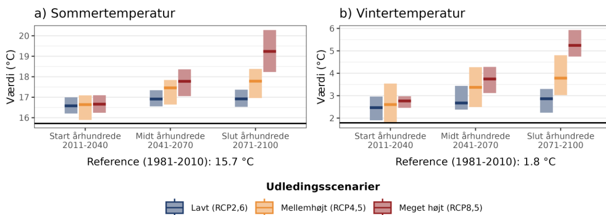
Figur 4. Fremtidens gennemsnitstemperatur for a) sommer (jun-aug) og b) vinter (dec-feb) under forskellige udledningsscenarier i Haderslev Kommune. Den sorte linje viser værdien for referenceperioden (1981-2010).
