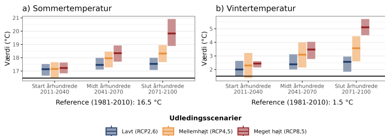
Figur 4. Fremtidens gennemsnitstemperatur for a) sommer (jun-aug) og b) vinter (dec-feb) under forskellige udledningsscenarier i Gladsaxe Kommune. Den sorte linje viser værdien for referenceperioden (1981-2010).
