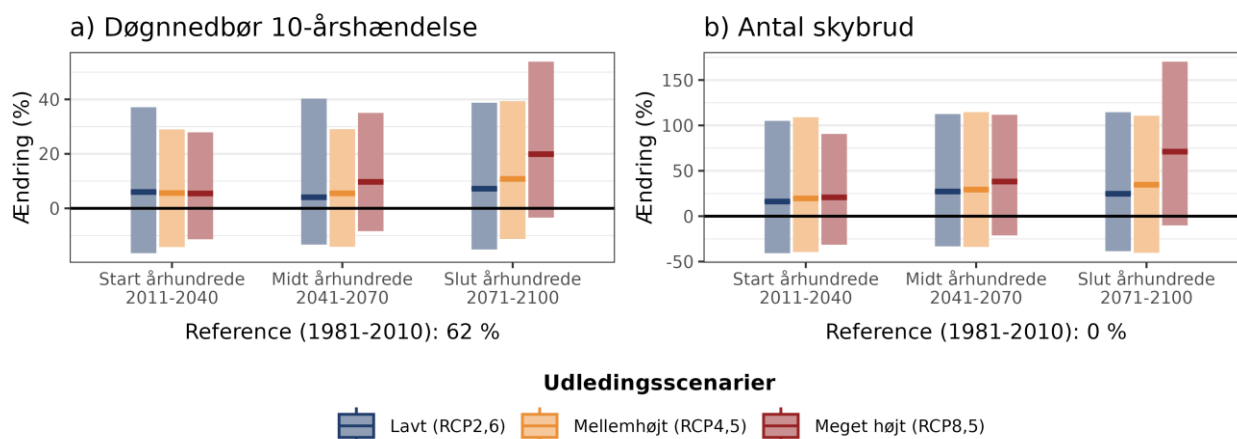
Figur 7. Procentvis ændring af a) 10-årshændelsen for døgnsnedbør og b) frekvensen af skybrud hen over året ift. 1981-2010 under forskellige udledningsscenarioer i Gladsaxe Kommune.
