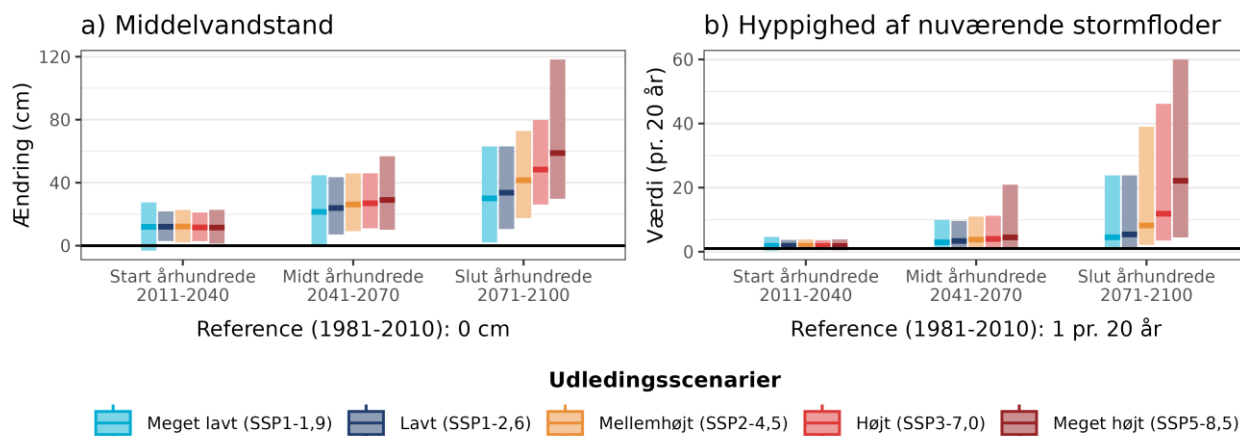
Figur 10. Fremtidens a) ændring i middelvandstand ift. referenceperioden 1981-2010 og b) hyppigheden af en nuværende 20-års stormflod for Isefjord under forskellige udledningsscenarier. Den sorte linje viser værdien for referenceperioden (1981-2010). Bemærk også at denne indikator maksimalt viser 60 stormfloder per 20 år, selv hvis de beregnede værdier bliver endnu højere.
