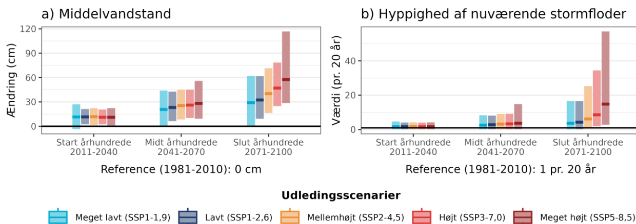
Figur 12. Fremtidens a) ændring i middelvandstand ift. referenceperioden 1981-2010 og b) hyppigheden af en nuværende 20-års stormflod for Roskilde Fjord under forskellige udledningsscenarier. Den sorte linje viser værdien for referenceperioden (1981-2010). Bemærk også at denne indikator maksimalt viser 60 stormfloder per 20 år, selv hvis de beregnede værdier bliver endnu højere.
