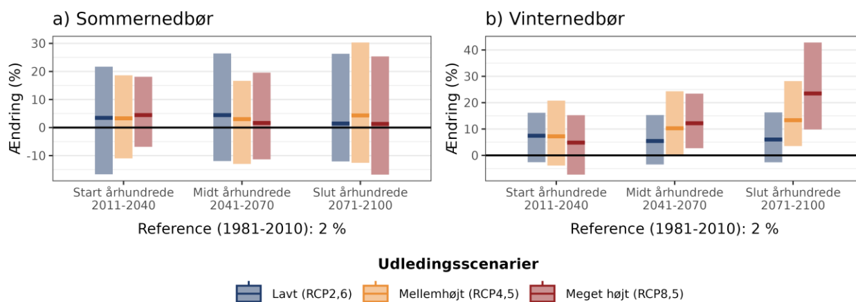
Figur 6. Procentvis ændring af middelnedbør a) om sommeren (jun-aug) og b) om vinteren (dec-feb) ift. referenceperioden 1981-2010 under forskellige udledningsscenarioer i Frederikssund Kommune.
