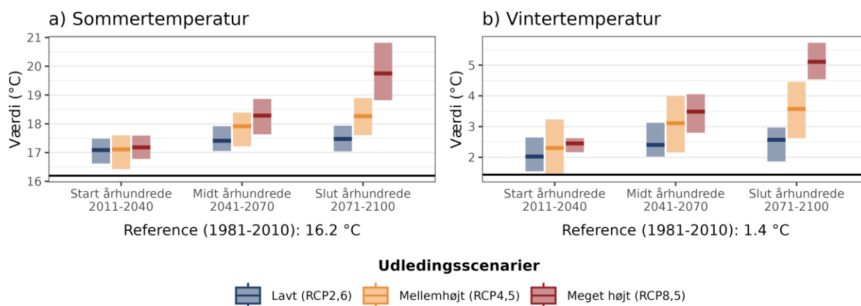
Figur 4. Fremtidens gennemsnitstemperatur for a) sommer (jun-aug) og b) vinter (dec-feb) under forskellige udledningsscenarier i Frederikssund Kommune. Den sorte linje viser værdien for referenceperioden (1981-2010).
