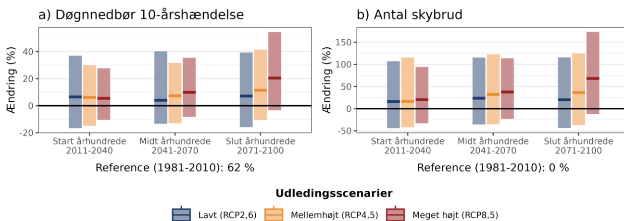
Figur 7. Procentvis ændring af a) 10-årshændelsen for døggnedbør og b) frekvensen af skybrud hen over året ift. 1981-2010 under forskellige udledningsscenarioer i Frederikssund Kommune.
