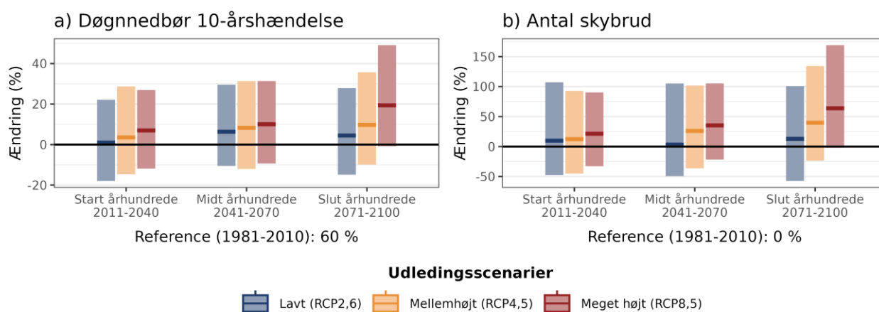
Figur 7. Procentvis ændring af a) 10-årshændelsen for døggnedbør og b) frekvensen af skybrud hen over året ift. 1981-2010 under forskellige udledningsscenarier i Frederikshavn Kommune.
