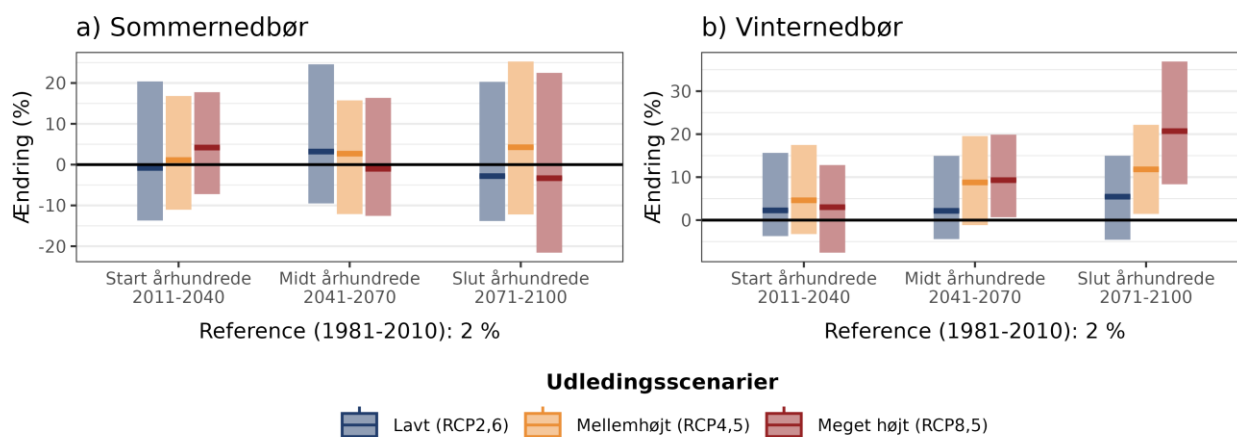
Figur 6. Procentvis ændring af middelnedbør a) om sommeren (jun-aug) og b) om vinteren (dec-feb) ift. referenceperioden 1981-2010 under forskellige udledningsscenarier i Frederikshavn Kommune.
