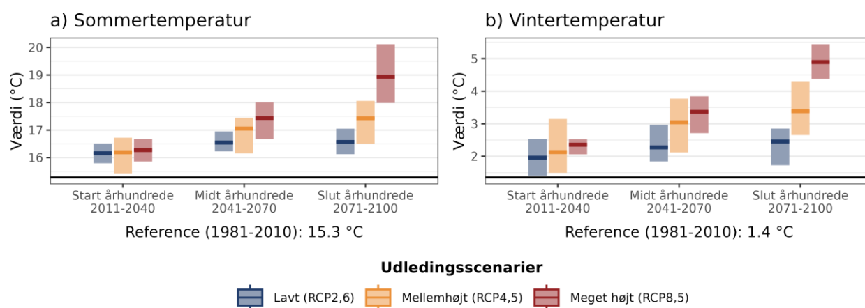
Figur 4. Fremtidens gennemsnitstemperatur for a) sommer (jun-aug) og b) vinter (dec-feb) under forskellige udledningsscenarier i Frederikshavn Kommune. Den sorte linje viser værdien for referenceperioden (1981-2010).
