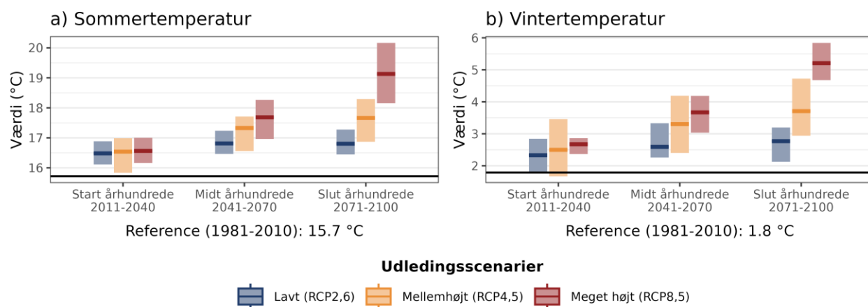
Figur 4. Fremtidens gennemsnitstemperatur for a) sommer (jun-aug) og b) vinter (dec-feb) under forskellige udledningsscenarier i Fredericia Kommune. Den sorte linje viser værdien for referenceperioden (1981-2010).
