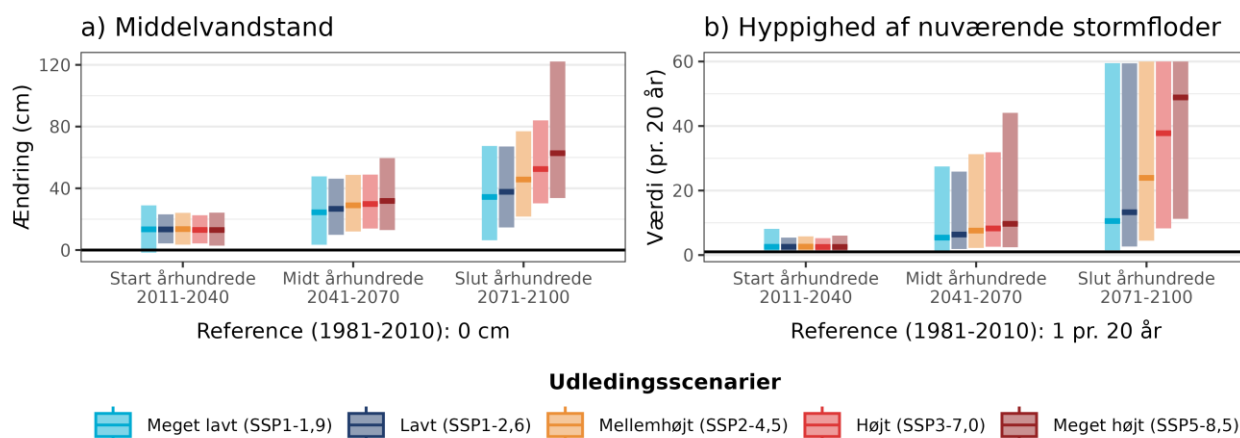
Figur 12. Fremtidens a) ændring i middelvandstand ift. referenceperioden 1981-2010 og b) hyppigheden af en nuværende 20-års stormflod for Lillebælt central under forskellige udledningsscenarier. Den sorte linje viser værdien for referenceperioden (1981-2010). Bemærk også at denne indikator maksimalt viser 60 stormfloder per 20 år, selv hvis de beregnede værdier bliver endnu højere.
