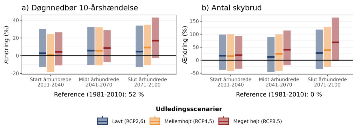
Figur 7. Procentvis ændring af a) 10-årshændelsen for døgnsnedbør og b) frekvensen af skybrud hen over året ift. 1981-2010 under forskellige udledningsscenarier i Fredericia Kommune.
