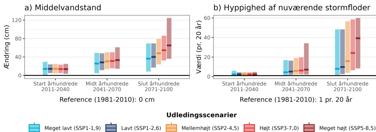
Figur 10. Fremtidens a) ændring i middelvandstand ift. referenceperioden 1981-2010 og b) hyppigheden af en nuværende 20-års stormflod for Lillebælt sydlig under forskellige udledningsscenarier. Den sorte linje viser værdien for referenceperioden (1981-2010). Bemærk også at denne indikator maksimalt viser 60 stormfloder per 20 år, selv hvis de beregnede værdier bliver endnu højere.
