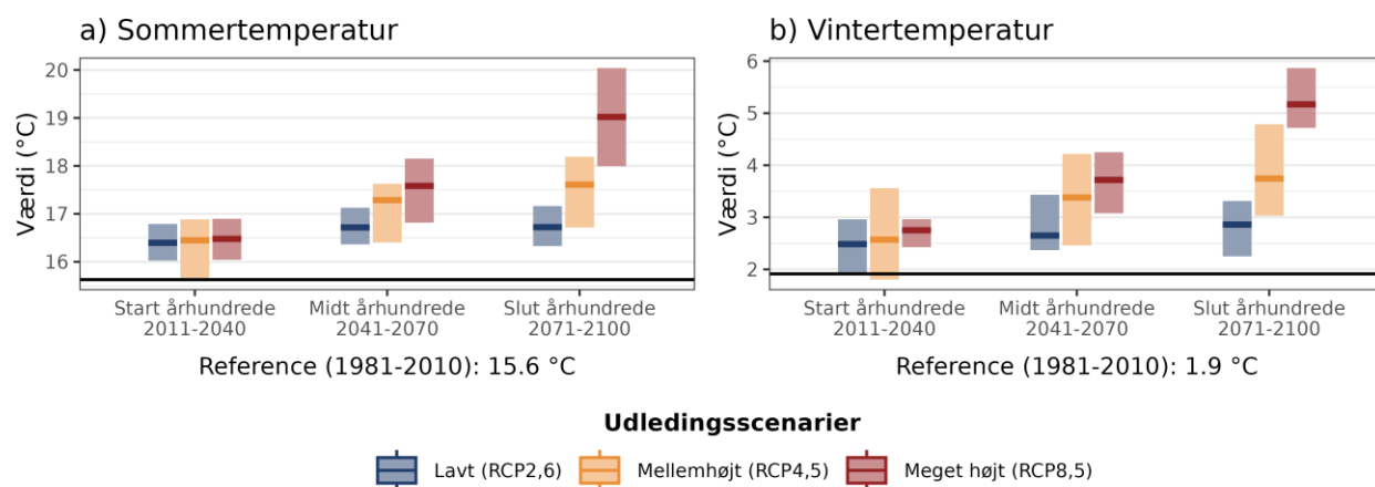
Figur 4. Fremtidens gennemsnitstemperatur for a) sommer (jun-aug) og b) vinter (dec-feb) under forskellige udledningsscenarier i Esbjerg Kommune. Den sorte linje viser værdien for referenceperioden (1981-2010).
