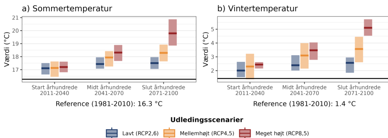
Figur 4. Fremtidens gennemsnitstemperatur for a) sommer (jun-aug) og b) vinter (dec-feb) under forskellige udledningsscenarier i Egedal Kommune. Den sorte linje viser værdien for referenceperioden (1981-2010).
