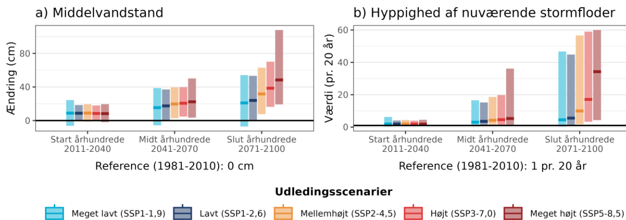
Figur 12. Fremtidens a) ændring i middelvandstand ift. referenceperioden 1981-2010 og b) hyppigheden af en nuværende 20-års stormflod for Kattegatkyst nordlige under forskellige udledningsscenarioer. Den sorte linje viser værdien for referenceperioden (1981-2010). Bemærk også at denne indikator maksimalt viser 60 stormfloder per 20 år, selv hvis de beregnede værdier bliver endnu højere.
