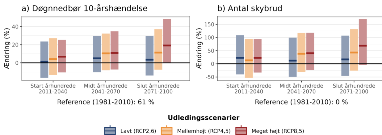
Figur 7. Procentvis ændring af a) 10-årshændelsen for døgnsnedbør og b) frekvensen af skybrud hen over året ift. 1981-2010 under forskellige udledningsscenarier i Aalborg Kommune.
