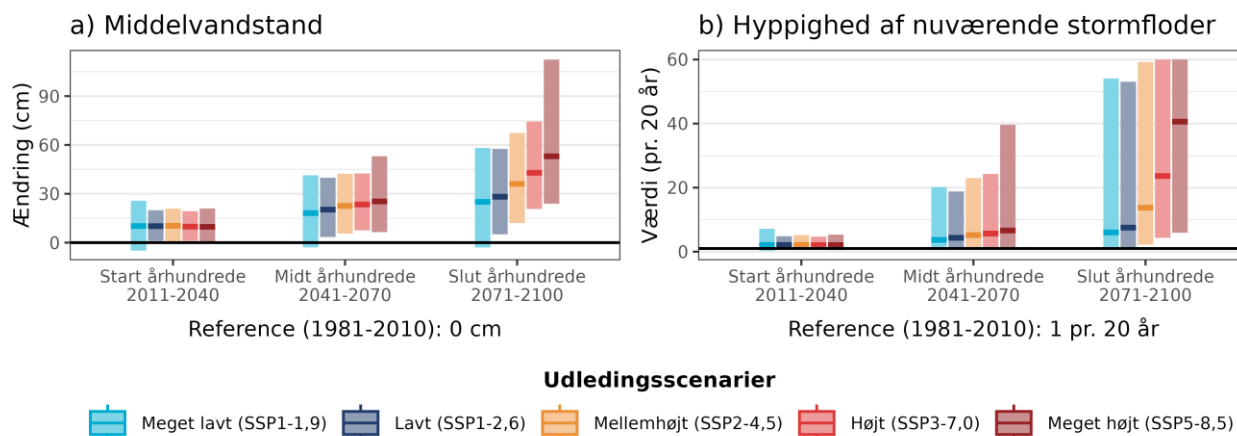
Figur 14. Fremtidens a) ændring i middelvandstand ift. referenceperioden 1981-2010 og b) hyppigheden af en nuværende 20-års stormflod for Ålborg Bugt under forskellige udledningsscenarier. Den sorte linje viser værdien for referenceperioden (1981-2010). Bemærk også at denne indikator maksimalt viser 60 stormfloder per 20 år, selv hvis de beregnede værdier bliver endnu højere.
