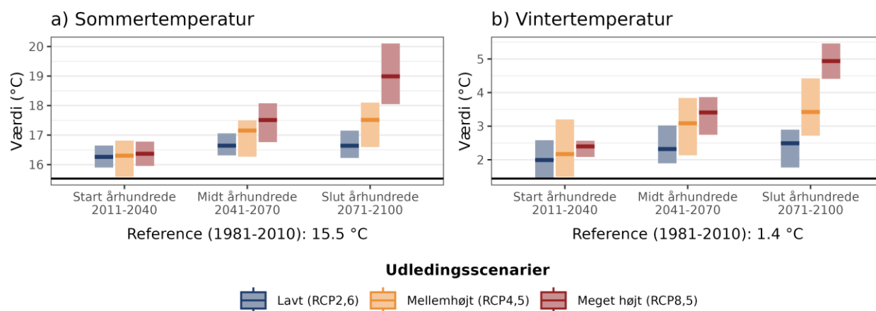
Figur 4. Fremtidens gennemsnitstemperatur for a) sommer (jun-aug) og b) vinter (dec-feb) under forskellige udledningsscenarier i Aalborg Kommune. Den sorte linje viser værdien for referenceperioden (1981-2010).
